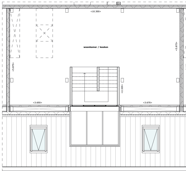
Plattegrond verdieping 04 1:50
