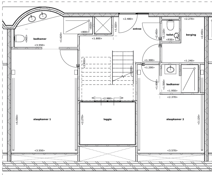
Plattegrond verdieping 03 1:50
